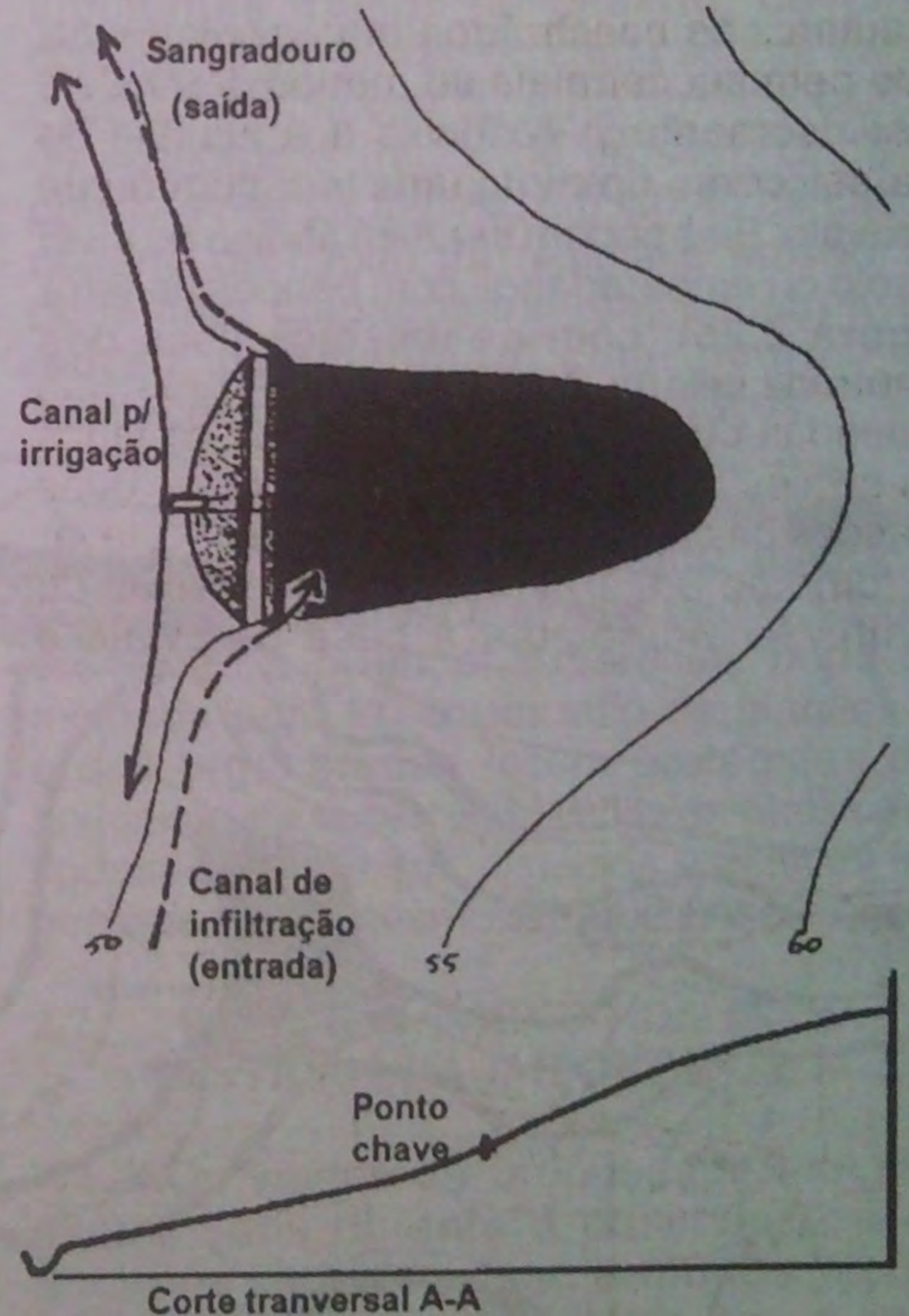
Figura 2.26 Açude de ponto chave. Se utilizados em séries não exigem ladrão, e o excesso é direcionado para o próximo açude e, eventualmente, para um córrego. Utilizado para sistemas de irrigação para encostas mais baixas.
