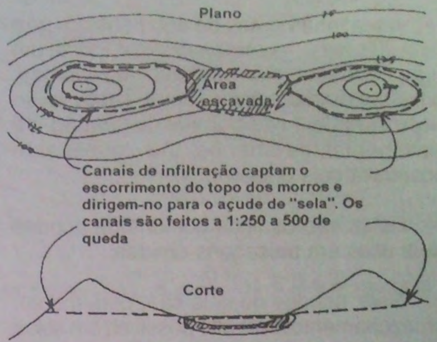
Figura 2.24 Açudes de sela são úteis para controle de fogo, vida silvestre e irrigação pequena. é a forma mais alta de açude em uma paisagem que coleta escoamento superficial (runoff)
