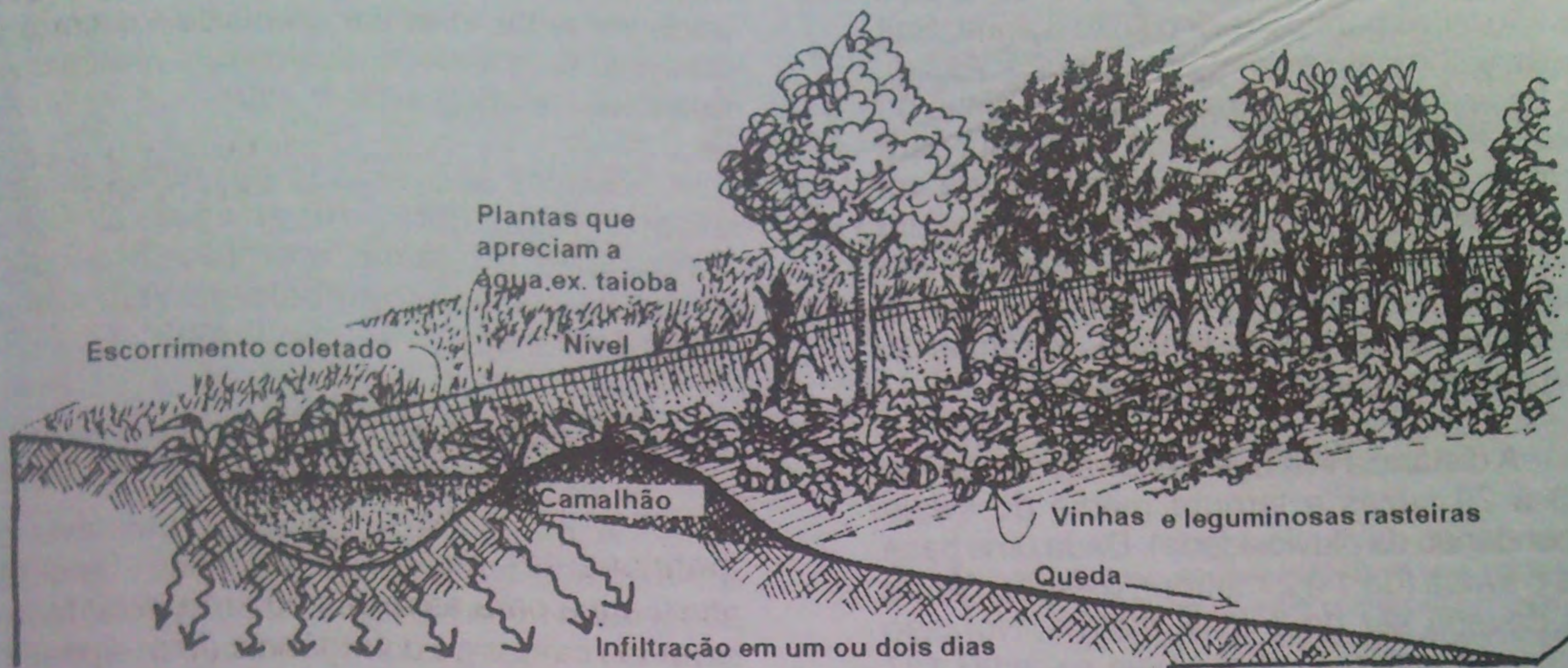
Figura 2.21 Canais de infiltração em curva de nível não permitem o movimento da água; primeiro armazenam e em seguida infiltram. Estes canais são plantados com árvores ou arbustos no lado interior.
