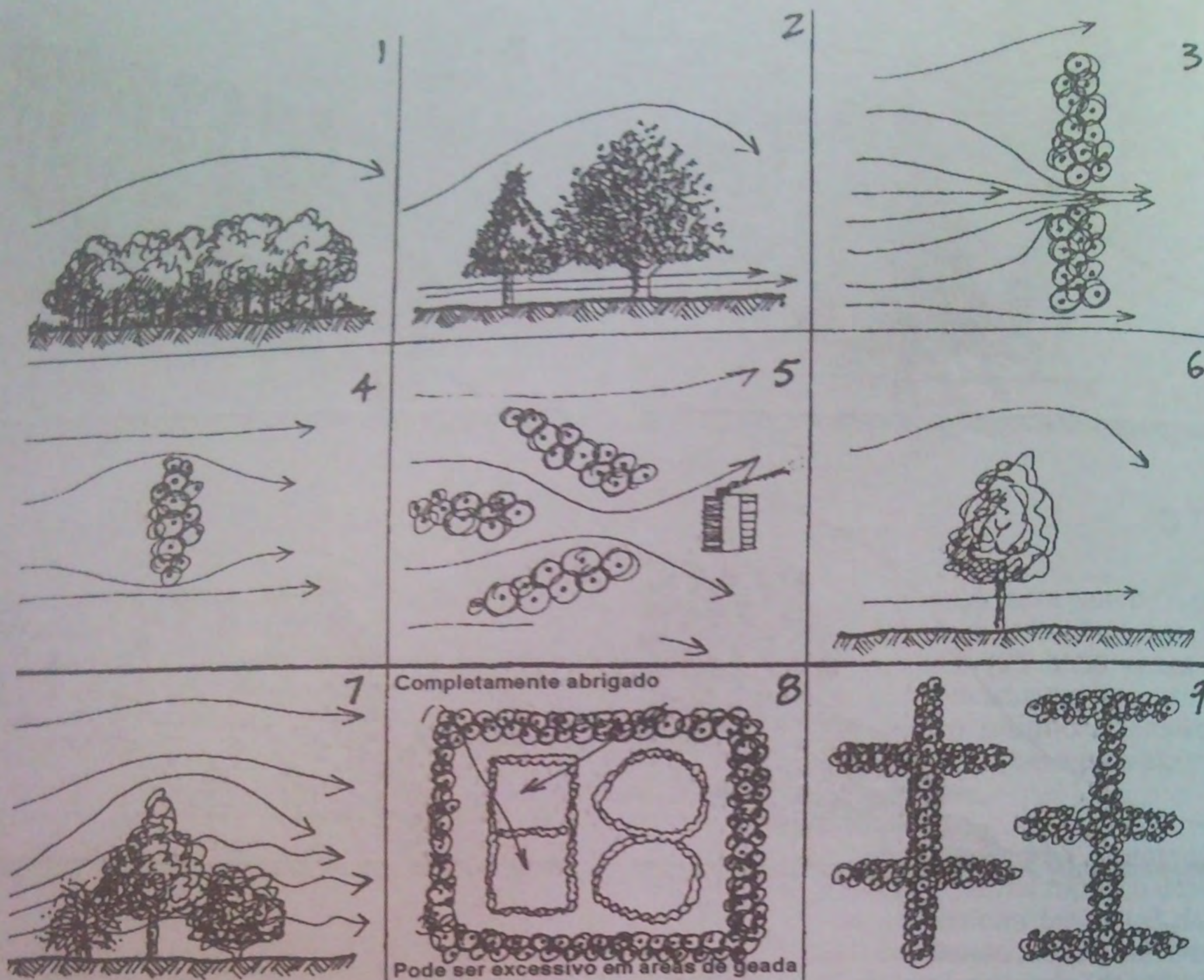
Figura 2.16 QUEBRA VENTOS QUE NÃO FUNCIONAM: (1) muito longo, (2) sem galhos baixos, acelera o vento, (3) lacunas aceleram o vento (efeito Venturi), (4) muito estreito, (5) não perpendicular ao vento, (6) somente uma carreira de árvores.
