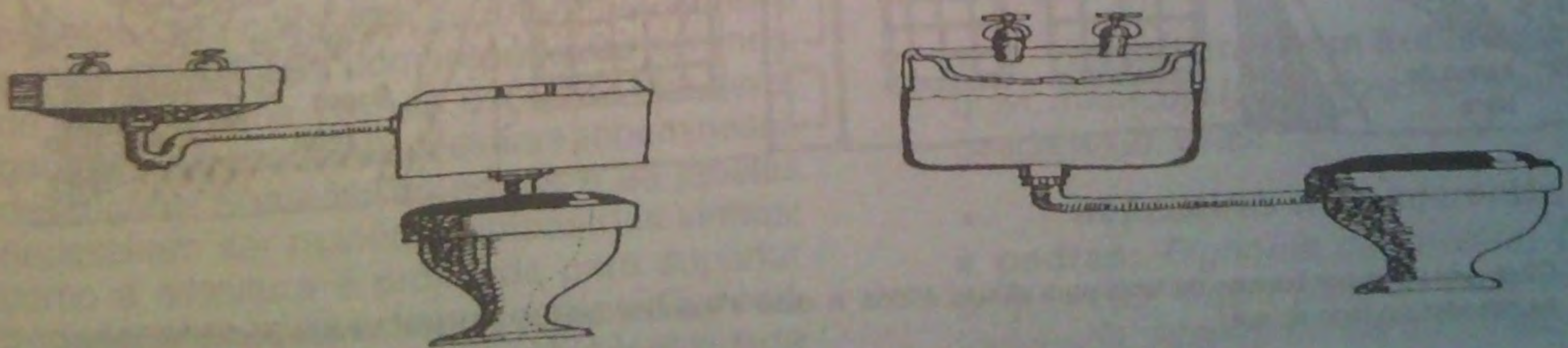
Figura 4.17 Formas para desviar a água da pia do banheiro e da lavanderia para o uso nos vasos sanitários.
