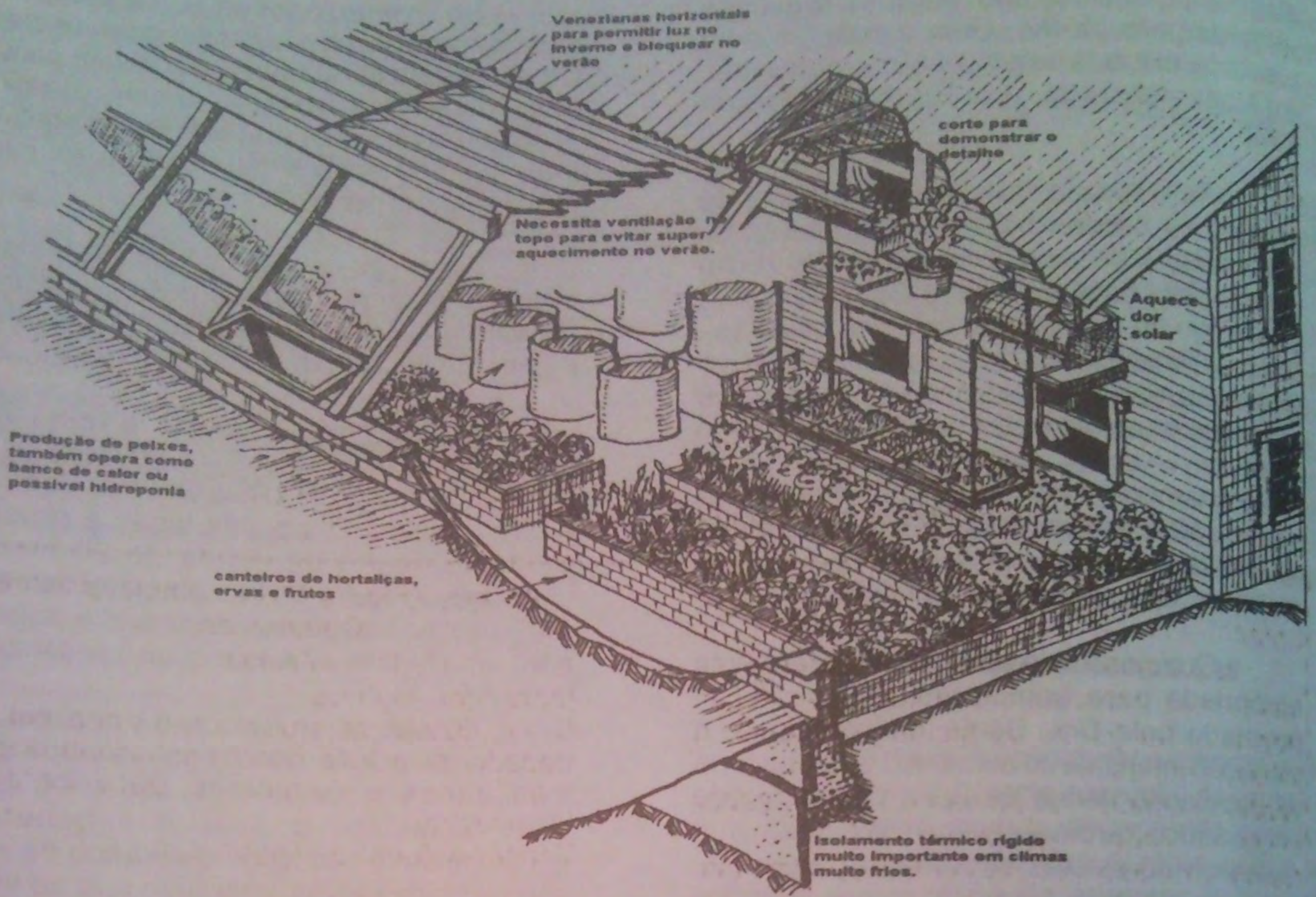
Figura 5.18 Estufa para peixes e produção de alimento em climas frios. Design do New Alchemy Institute: Bioshelter.
