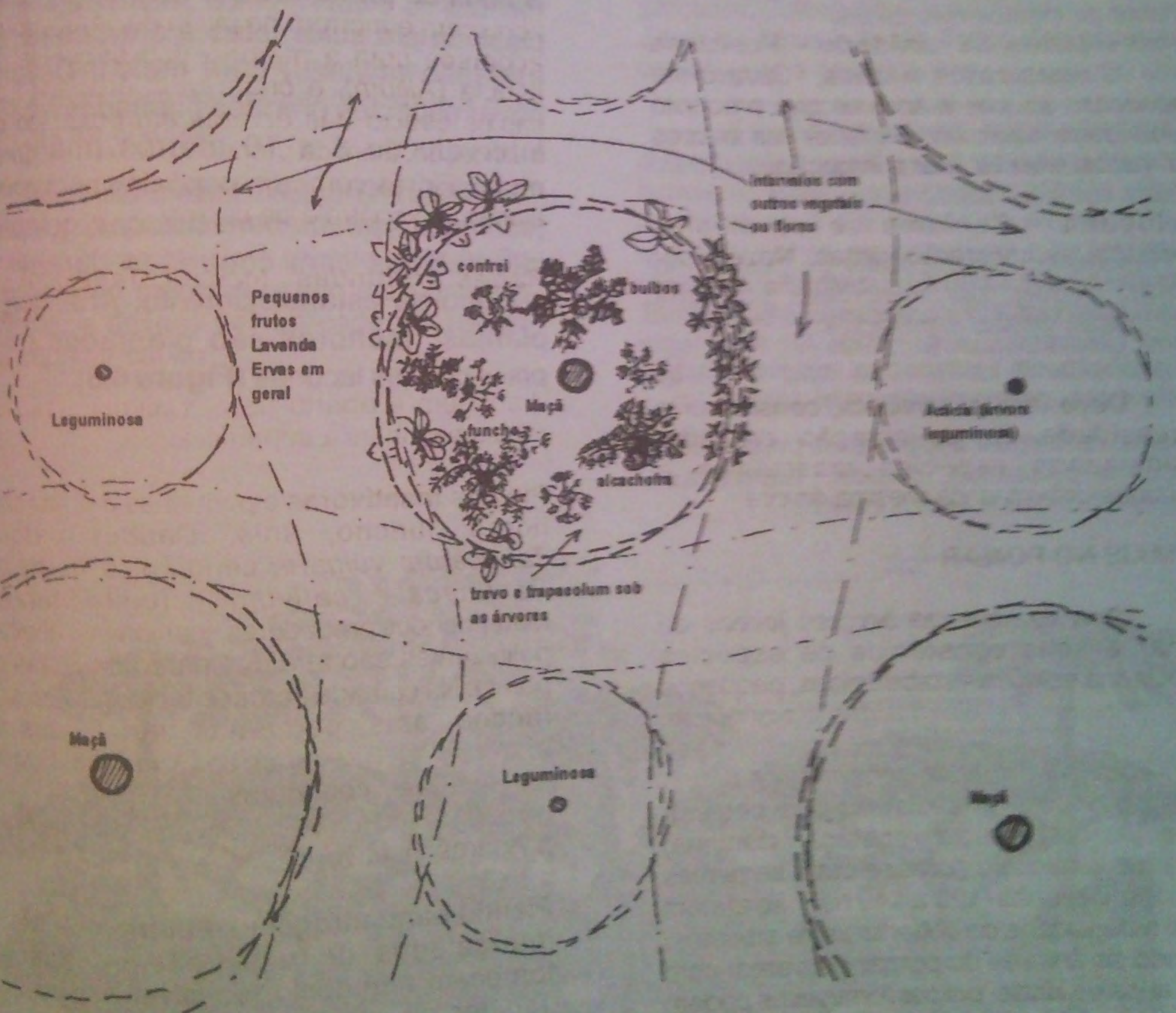
Figura 6.2 Consórcio idealizado para um pomar de macieiras. Árvores leguminosas são podadas na altura do peito para mulch; Flores perenes e anuais ajudam no controle de insetos; o capim é eliminado com confrei e ervas.
