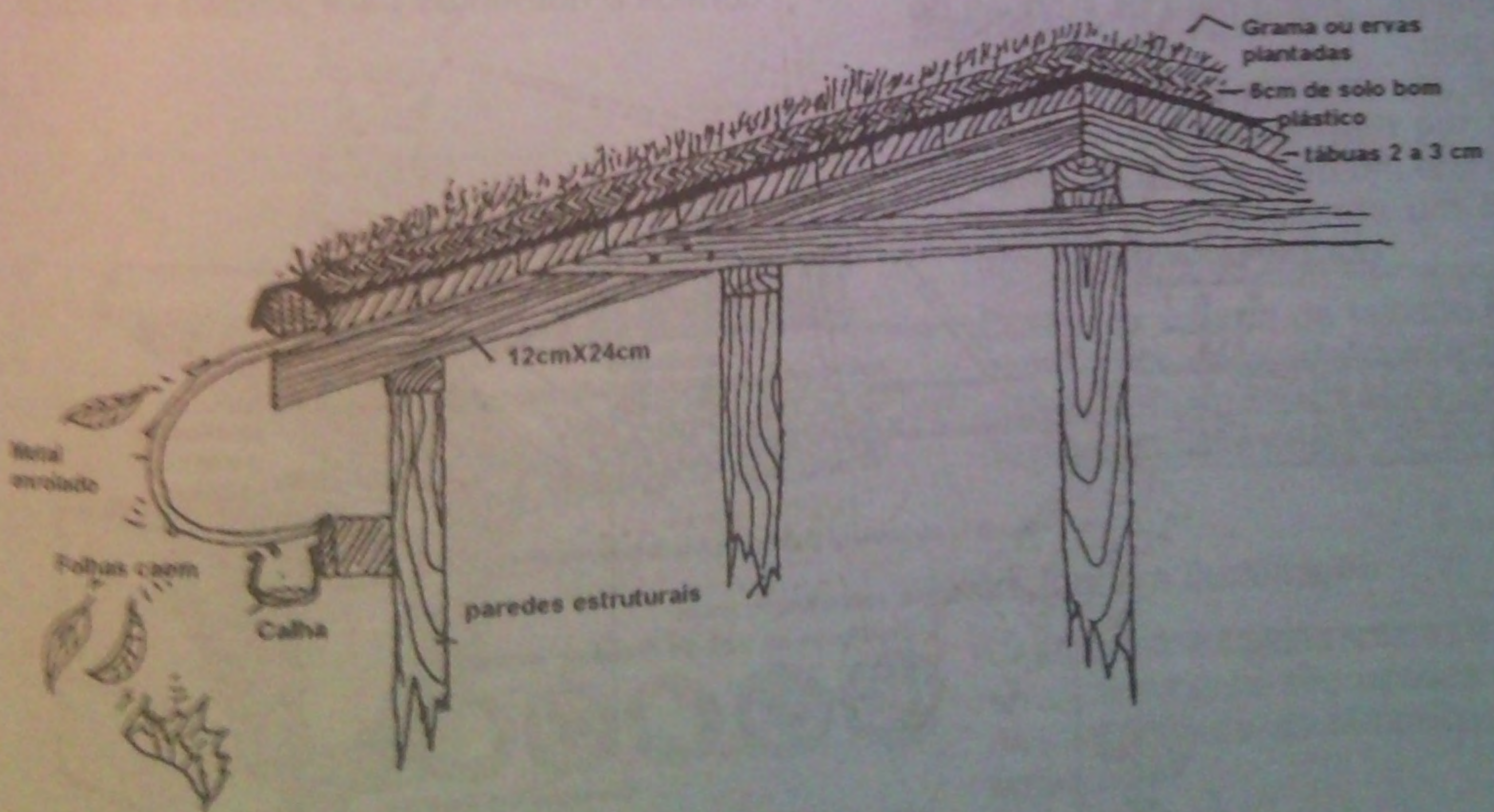
Figura 4.21 Construção de telhado de grama.
