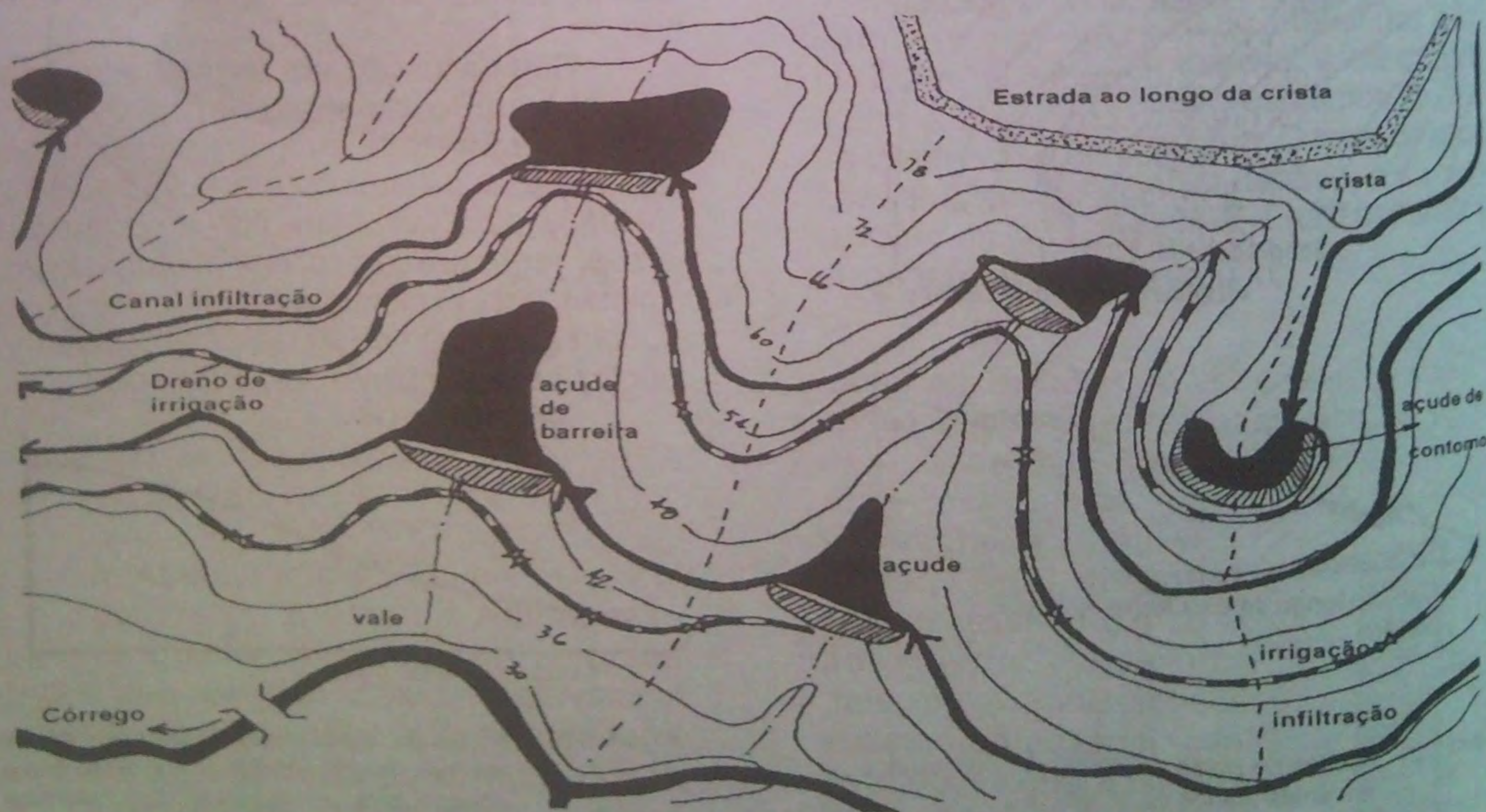
Figura 2.27 - O sistema de linha chave de P.A. Yeomans, oferece irrigação a prova de secas para fazendas. Com manutenção e custos de operação muito baixos, seus livros abordam o design para eficiência hidráulica para fazendas, acessos, cinturões de árvores, melhoria do solo e armazenamento de água criativos.
