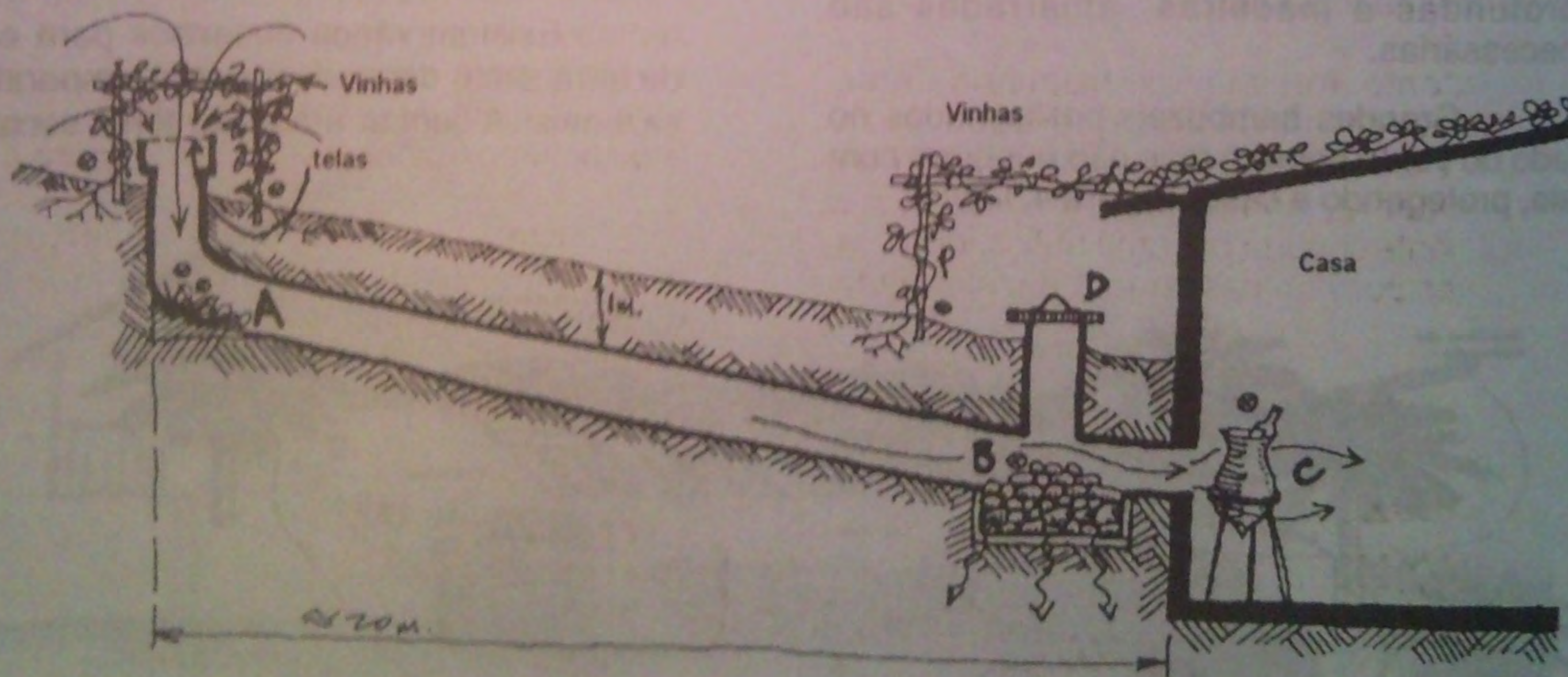
Figura 4.15 Túnel cria fluxo de ar frio e úmido em casas no deserto. Inclinado para a casa, o túnel tem uma entrada sombreada, uma cama de rocha úmida e um pote de água na saída. Comprimento: 20 metros.
