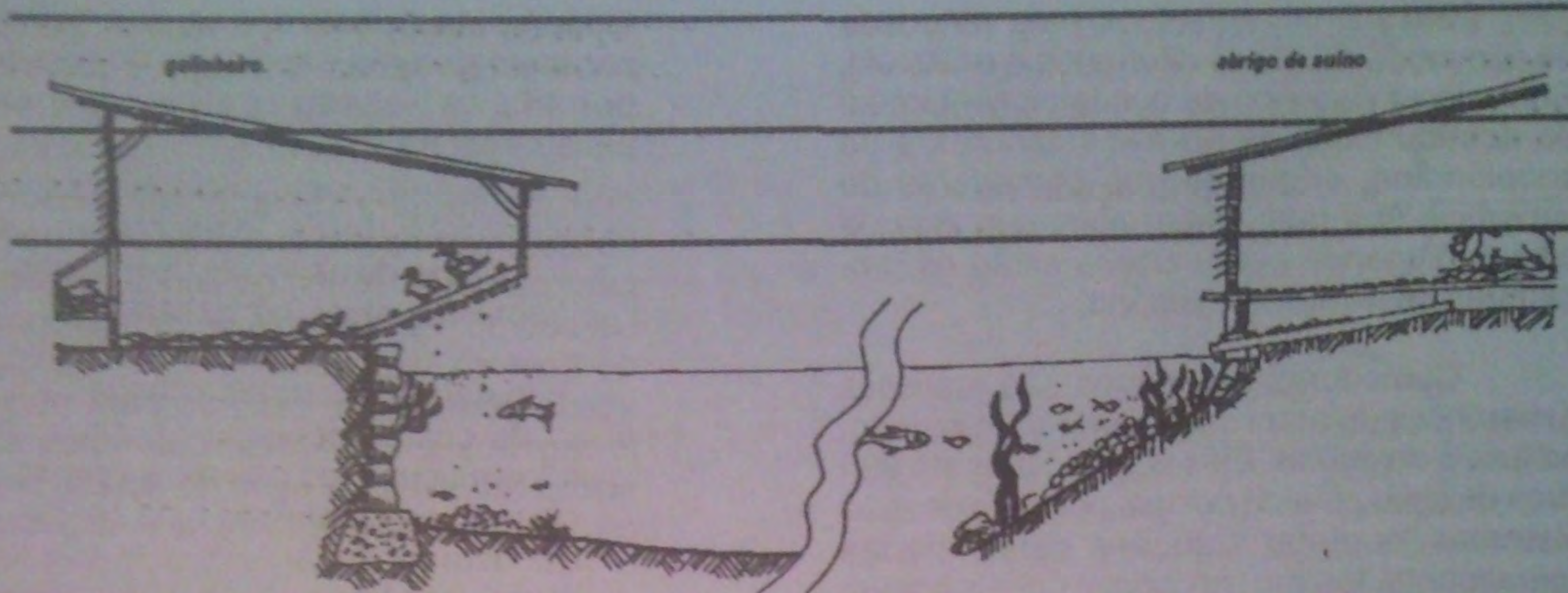
Figura 7.21 Utilizado amplamente na Ásia, estercos animais são usados para fertilizar os tanques. Isto é facilmente alcançado se os abrigos são localizados sobre o tanque. Pisos devem ser gradeados de forma que o esterco caia na água.
