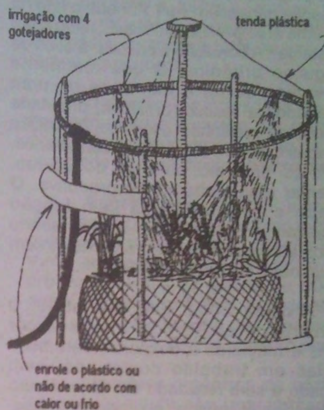
Figura 5.17c Canteiro circular com proteção plástica.
