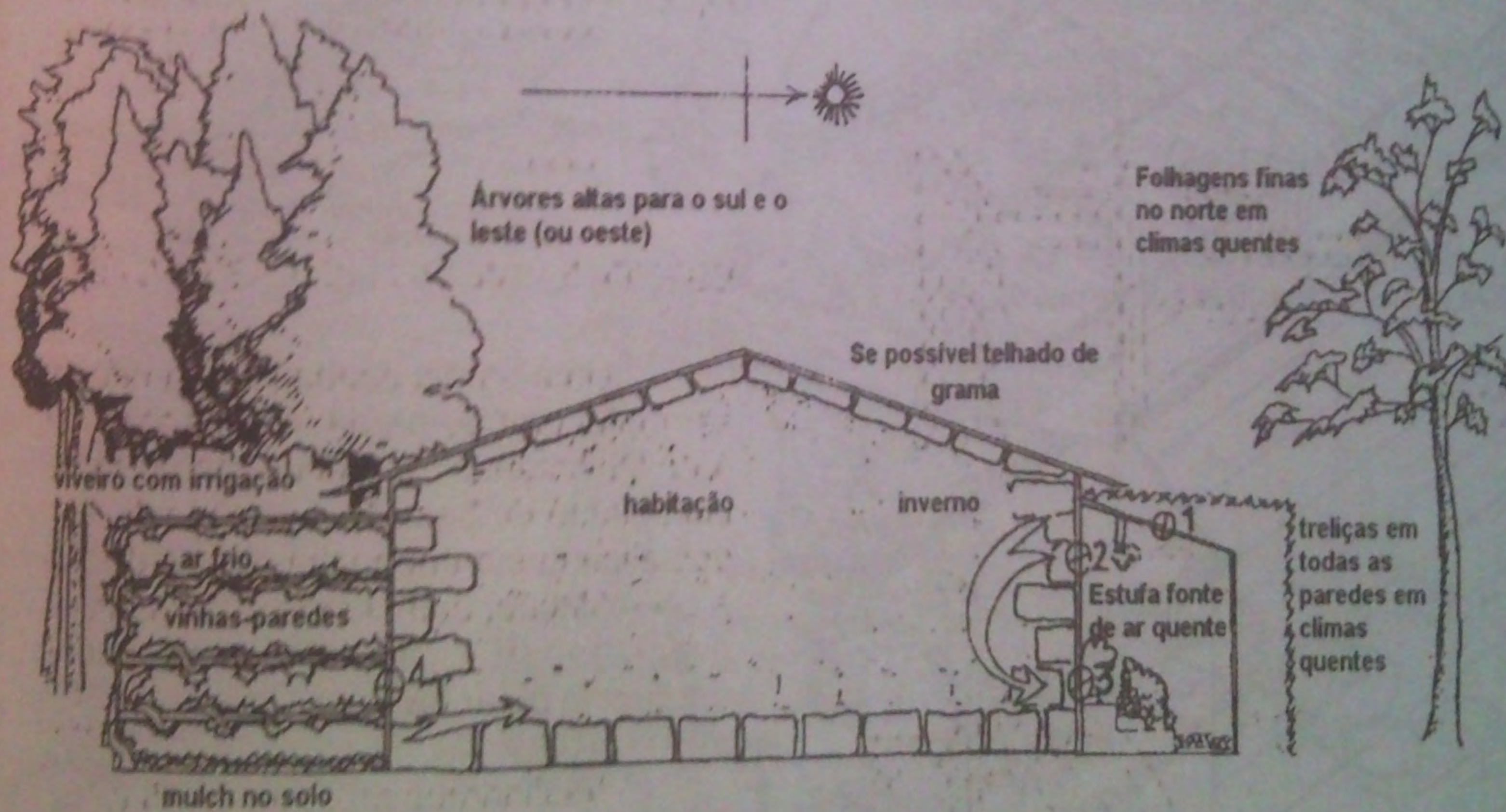
Figura 4.9 Ar frio circula do viveiro para a casa, sugado pela estufa. Vinhas caducifólias (uvas) estão no lado do sol, enquanto que vinhas perenifólias estão no lado da sombra.
