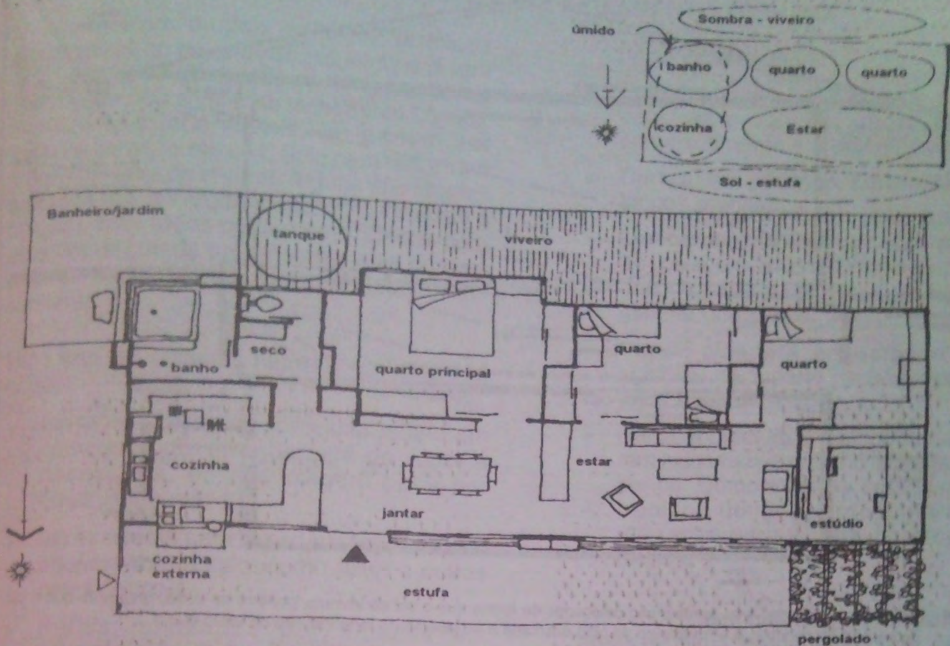
Figura 4.5 Design de uma casa para clima temperado. Apresenta um desenho dos quartos para o lado frio da casa, e as áreas de estar no lado do sol para aquecimento no inverno. A cozinha e o banheiro partilham os canos de água e deveriam ser posicionados juntos
