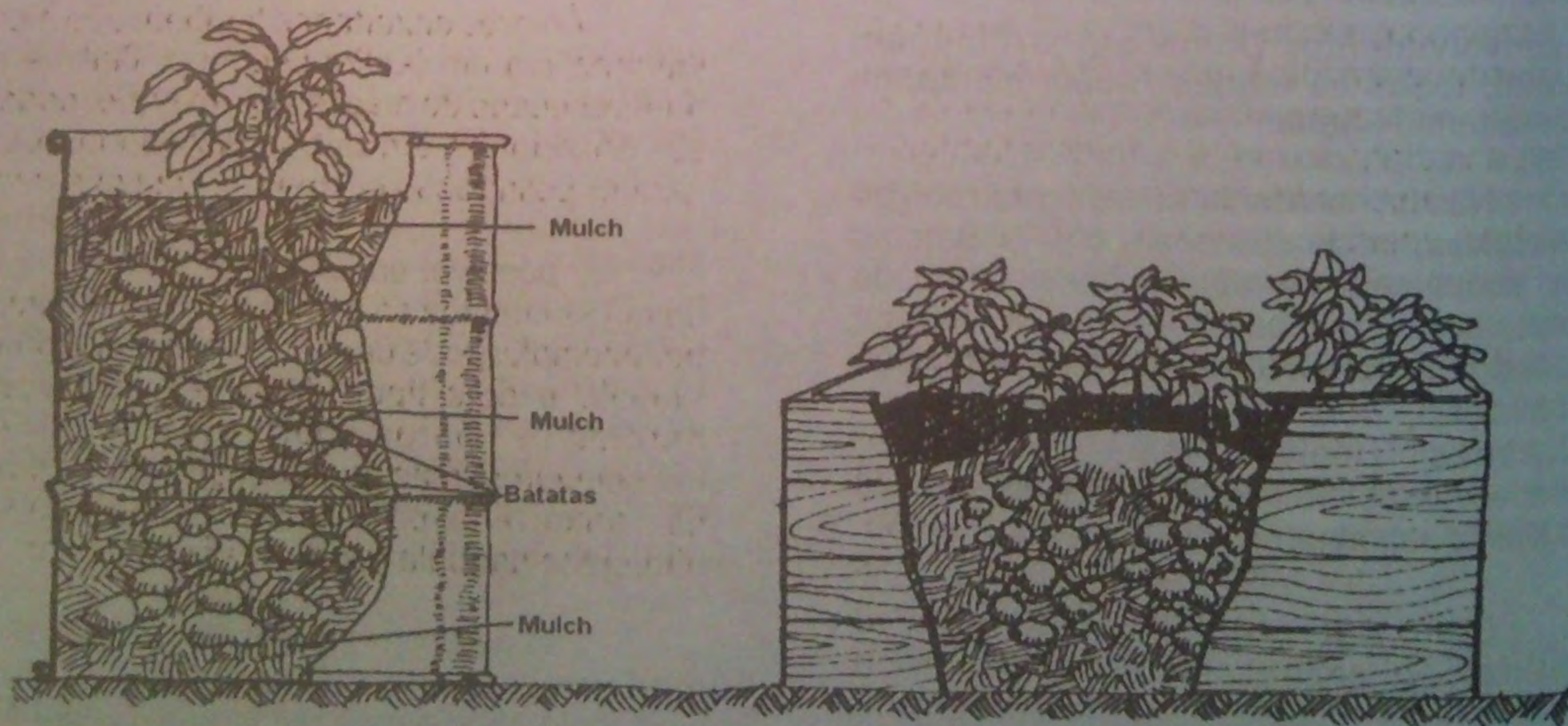
Figura 5.13 Caixas para batatas. Esquerda: tambor de 200 litros com o nível de mulch elevado a medida que as plantas cresçam. Direita: caixa construída em seções adicionais quando necessário.
