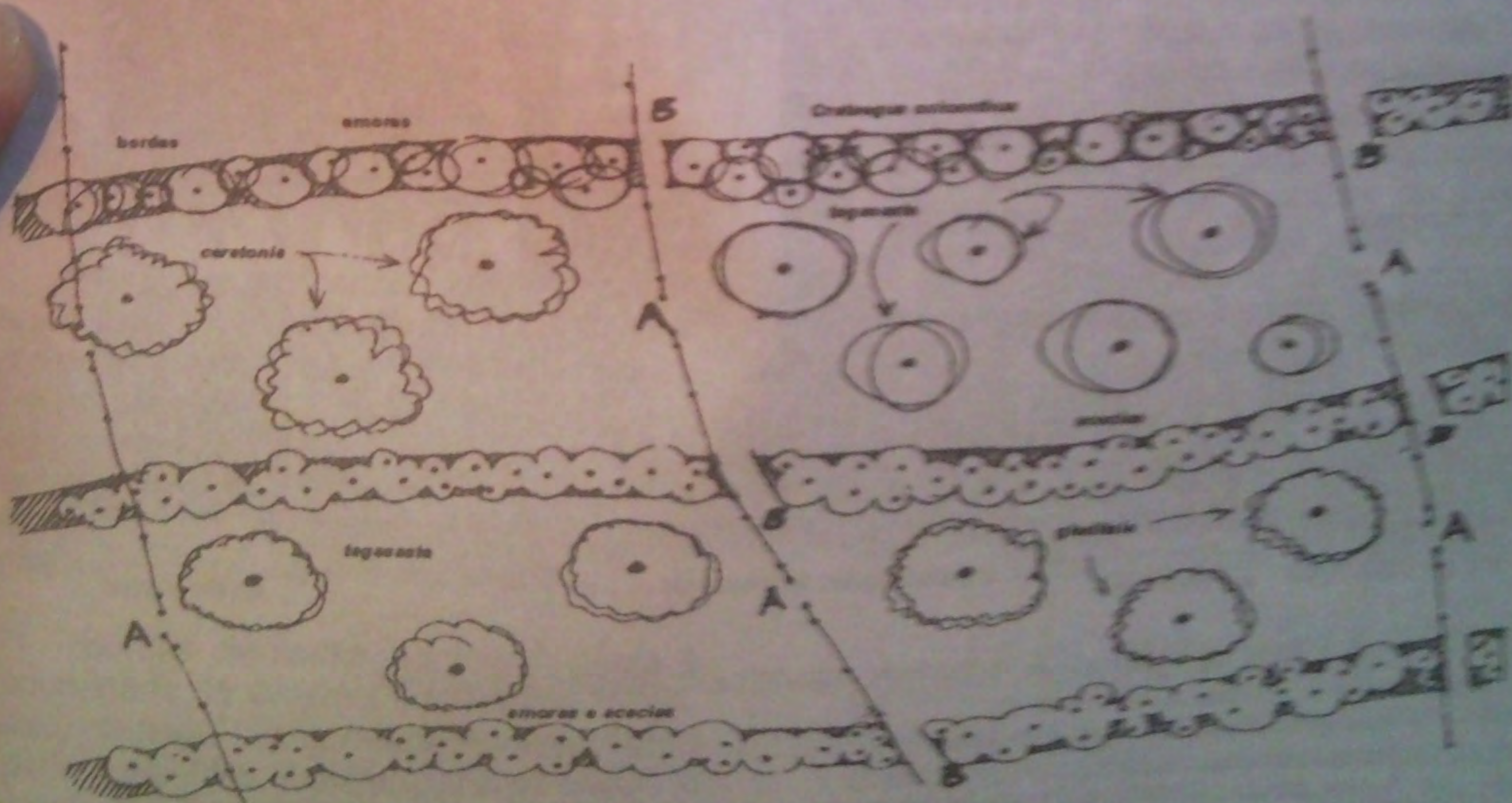
Figura 7.16 Cercados rotativos com cercas vivas entre as faixas cercadas em curva de nível. O gado pode ser movido ao longo das curvas de nível pelos portões B. Estes podem ser semeados com forrageiras. Uma vez estabelecidos, as cercas vivas podem acomodar visitas periódicas do gado. Portões e cercas devem ser sempre localizados nas cristas (não nos vales) para prevenir a erosão que ocorre nestas áreas muito utilizadas. Adaptado de um desenho de Tony Gilfedder.
